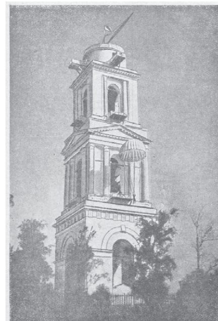
Рис. 5. Колокольня церкви, оборудованная под вышку Ржевского аэроklubом. Общая высота - 65 м, высота третьей рабочей площадки - 29 м, второй площадки - 42 м и первой - 24 м. Вышка имеет 9 площадок, выходящих на три стороны. Длина канатки - 12,1 м.
